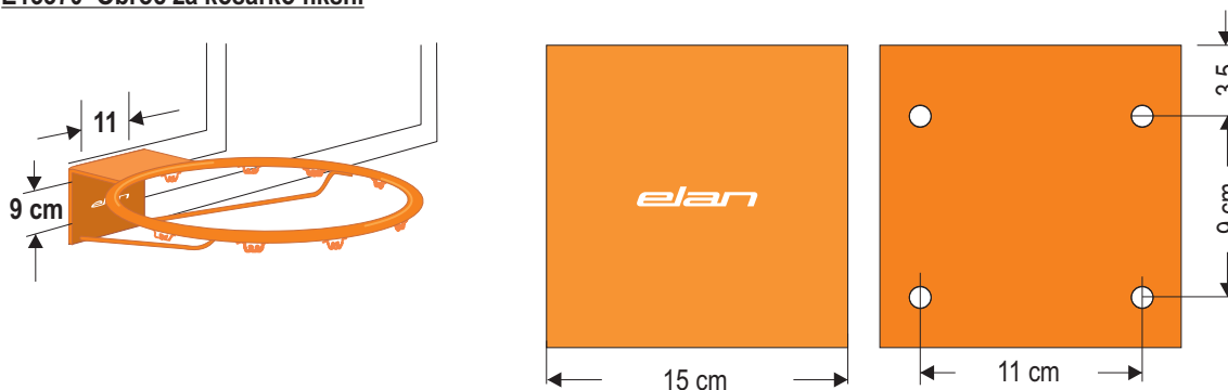
E13370 Obroč za košarko fiksni
