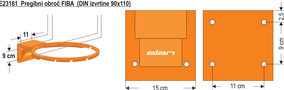
E23161 Pregibni obroč FIBA (DIN izvrtine 90x110)
