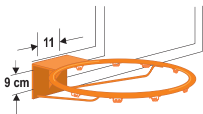
E13371 Obroč za košarko fiksni 263
